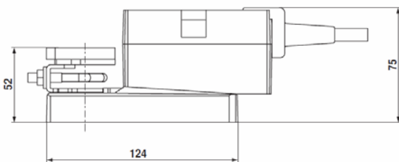
寸法図 (単位mm)
