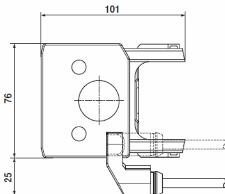
寸法図 (単位 mm)
